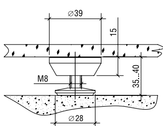
Опора Н40 М регулируемая (СК34) Support adjustable art. H 40 M (СК34)
