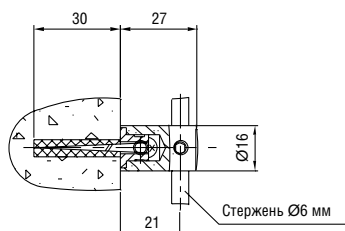
Узел СТ 14.11 Fastening unit RS 14.11
