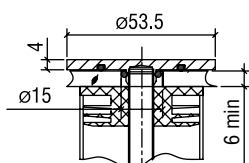
Заглушка H55 Gag art. H55
