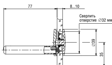
Держатель 7.107 Holder art. 7.107
