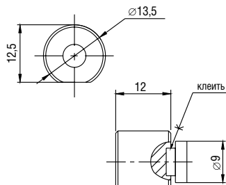
Защелка магнитная (СК43) Magnetic catch art. CK43
