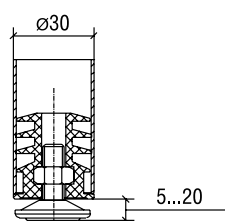
Опора П30 регулируемая Support adjustable art. P30
