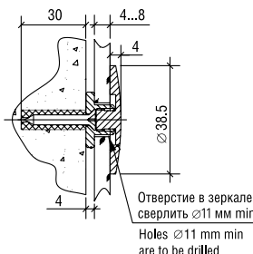
Держатель 5.10/5.10D Holder art. 5.10/5.10D
