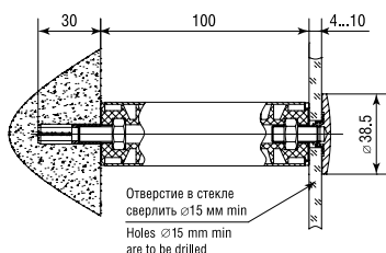
Шайба дистанционная 11.01 Distant washer 11.01
