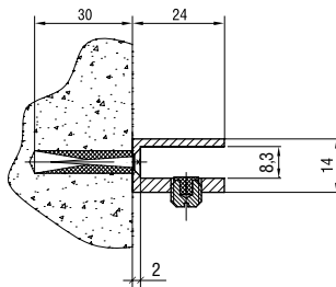
Кронштейн 3.21 M Bracket art. 3.21 M
