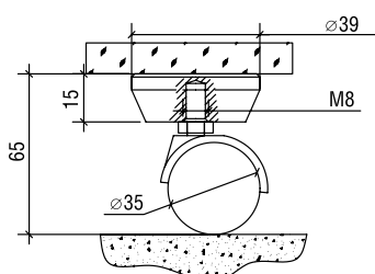
Опора Н40 Р с роликом (СК19) Support with a roller art. H40 R (СК19)
