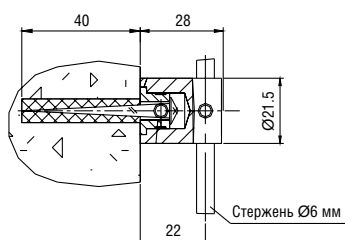
Узел СТ 14.11 Fastening unit RS 14.11
