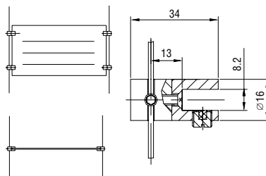
Кронштейн ТС 5.01 Bracket RS 5.01
