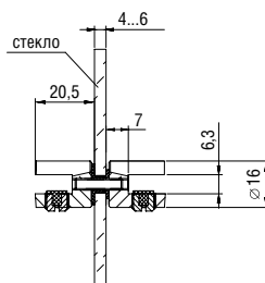
Кронштейн 4.06 Bracket 4.06
