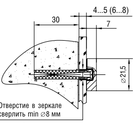
Держатель 5.12 H; D=22 мм Holder art. 5.12 H; D=22 mm
