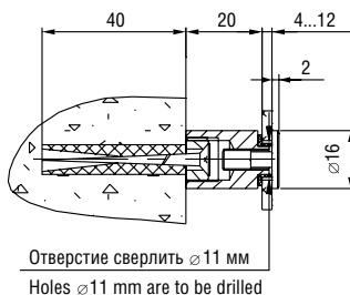
Держатель 5.43N Holder art. 5.43N
