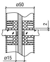
Узел разрыва P50 Break unit art. P50
