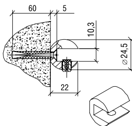
Кронштейн 3.09M; L=24 mm Bracket art. 3.09M; L=24 mm
