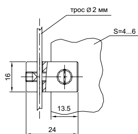
Держатель ТС 4.01 Holder RS 4.01
