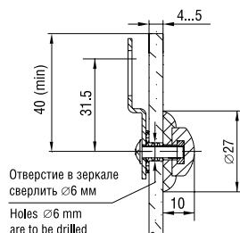
Подвеска 2.13 Clip art. 2.13
