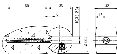
Кронштейн 3.22 Bracket art. 3.22
