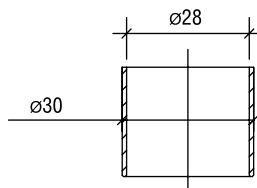
Труба П30 Tube art. P30
