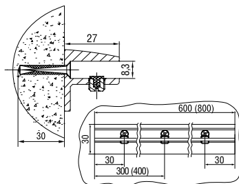
Матрица светодиодная LED matrix
