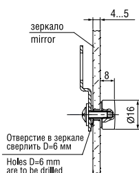
Подвеска 2.15 Clip art. 2.15
