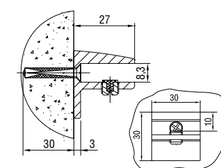
Кронштейн 3.08; L=30 мм Bracket art. 3.08; L=30 mm
