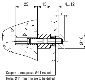
Держатель 5.33 Holder art. 5.33
