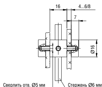
Держатель СТ 14.04 Holder RS 14.04
