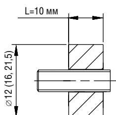
Шайба дистанционная 11.01 Distant washer 11.01
