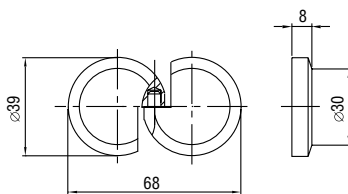
Петля Cristallo Hinge Cristallo
