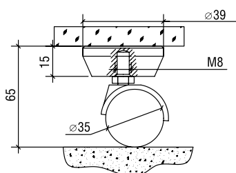
Опора КД40 Р с роликом (СК18) Support with a roller art. KD40 R (СК18)
