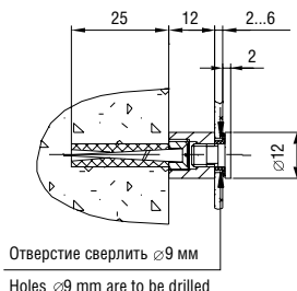
Держатель 5.43H Holder art. 5.43H
