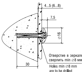
Держатель 5.01H/5.01Д; D=16 мм Holder art. 5.01H/ 5.01Д; D=16 мм
