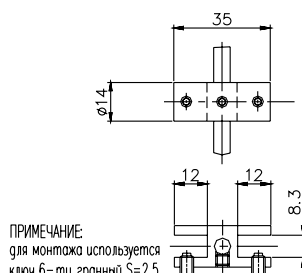
Кронштейн СТ 22.10 (Amsterdam) Bracket RS 22.10 (Amsterdam)
