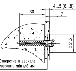
Держатель 5.12 M; D=22 мм Holder art. 5.12 M; D=22 mm
