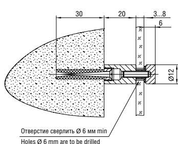
Держатель 5.16M CM, ЧМ Holder art. 5.16M SM, BM
