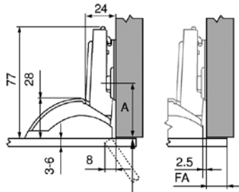
Петля Cristallo Hinge Cristallo
