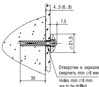
Держатель 5.01H/5.01Д; D=22 мм Holder art. 5.01H/5.01Д; D=22 мм
