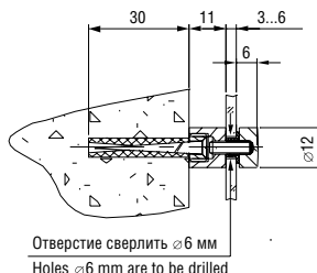
Держатель 5.16 Holder art. 5.16
