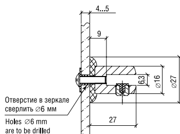
Кронштейн 2.01 М Bracket art. 2.01 М
