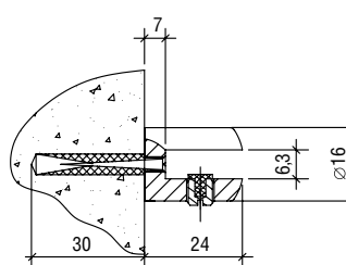
Кронштейн 3.06 M Bracket art. 3.06 M
