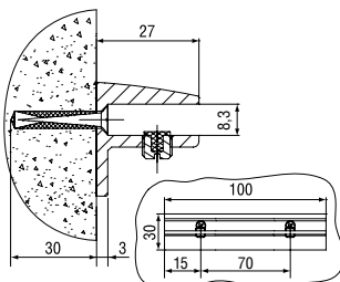
Кронштейн 3.08; L=100 mm Bracket art. 3.08; L=100 mm
