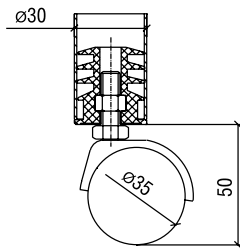
Опора П30 колесная Roller support unit art. P30
