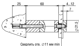
Держатель 5.33 Holder art. 5.33
