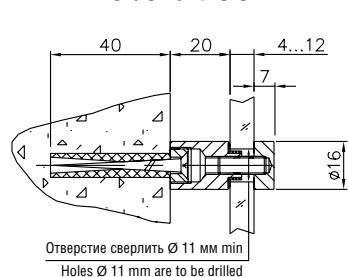
Держатель 5.37 Holder art. 5.37
