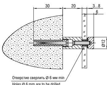
Держатель 5.16M Holder art. 5.16M
