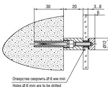
Держатель 5.16H Holder art. 5.16H
