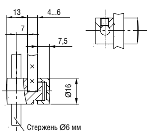
Держатель СТ 14.10 Holder RS 14.10
