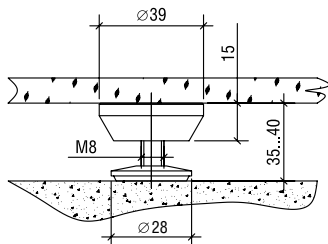
Опора КД 40 М регулируемая (СК33) Support adjustable art. KD 40 M (СК33)
