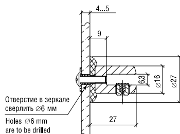
Кронштейн 2.03 М Bracket art. 2.03 М
