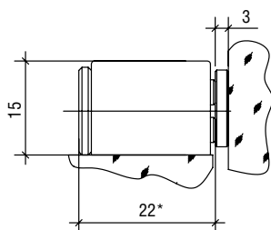
Защелка магнитная (СК28) Magnetic catch art. CK28
