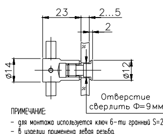
Держатель СТ 22.12 (Burgas) Holder RS 22.12 (Burgas)
