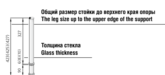
Модель 3 Model 3
