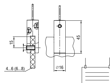
Кронштейн ТС 5.04 Bracket RS 5.04
