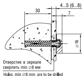
Держатель 5.12; D=16 мм Holder art. 5.12; D=16 mm
