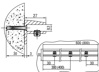
Кронштейн 3.09M; L=24 mm Bracket art. 3.09M; L=24 mm
