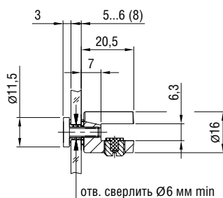
Кронштейн 4.06 Bracket 4.06
