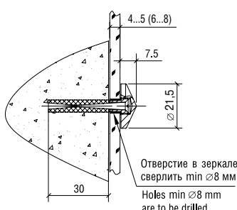
Держатель 5.01H/5.01Д; D=22 мм Holder art. 5.01H/5.01Д; D=22 мм
