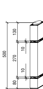
Модель 5-3 Model 5-3
