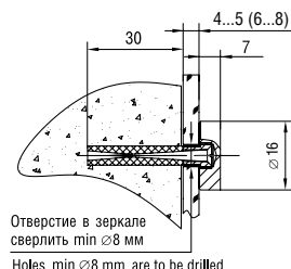
Держатель 5.12 H; D=16 мм Holder art. 5.12 H; D=16 mm
