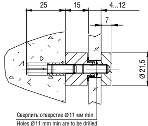
Держатель 5.33 Holder art. 5.33
