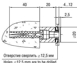
Держатель 5.16M Holder art. 5.16M
