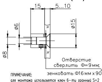
Держатель 21.05 (Ufa) Holder art. 21.05 (Ufa)
