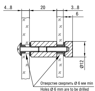
Держатель 5.37 Holder art. 5.37
