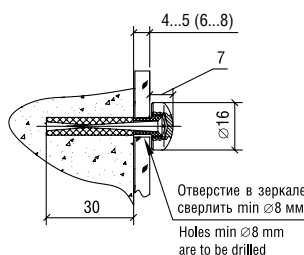
Держатель 5.10/5.10D Holder art. 5.10/5.10D
