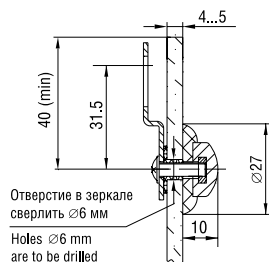
Подвеска 2.11 Clip art. 2.11
