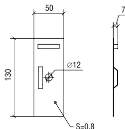
Пластина Тип 1 оцинкованная Zinc-coated Plate Type 1
