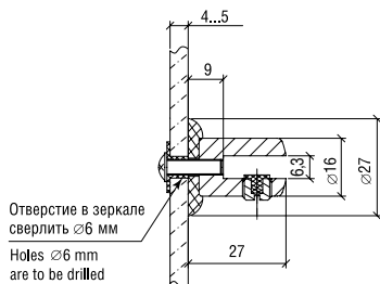
Кронштейн 2.02 М Bracket art. 2.02 М
