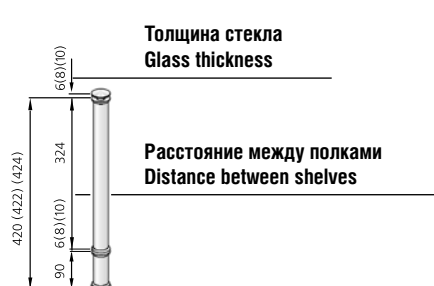
Модель 3 Model 3
