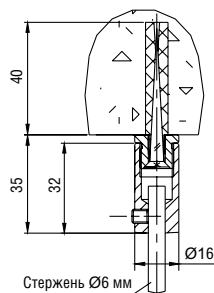
Узел СТ 14.02 Fastening unit RS 14.02
