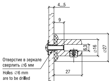
Кронштейн 2.05 М Bracket art. 2.05 М
