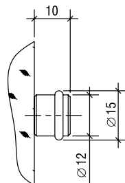
Упор (Полкодержатель) Support (Shelf-holder)
