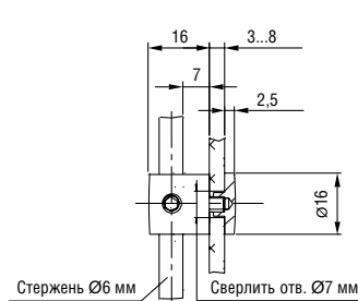
Держатель СТ 14.12 Holder RS 14.12
