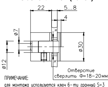
Держатель 21.04 (Zurich) Holder art. 21.04 (Zurich)
