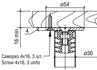
Фланец П30 под саморез Flange art. P30 with screw
