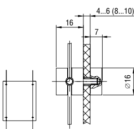
Держатель ТС 4.01 Holder RS 4.01
