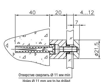
Держатель 5.38 Holder art. 5.38
