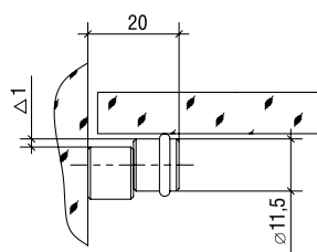
Полкодержатель эксцентриковый (СК16) Eccentric Shelf-holder art. CK16
