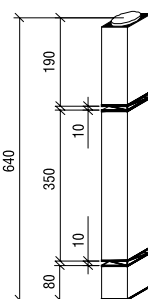
Модель 5-2 Model 5-2
