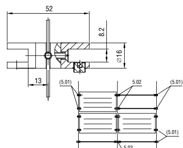
Кронштейн ТС 5.03 Bracket RS 5.03
